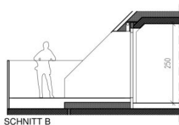
SCHNITT B
