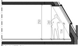
SCHNITT B3
