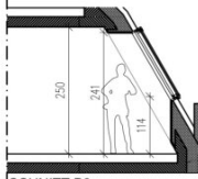
SCHNITT B3
