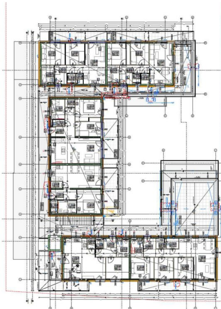
Grundriss 2. Obergeschoß
