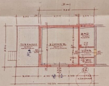
GRUNDRISS
