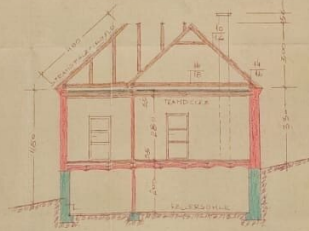
Schnitt ab
