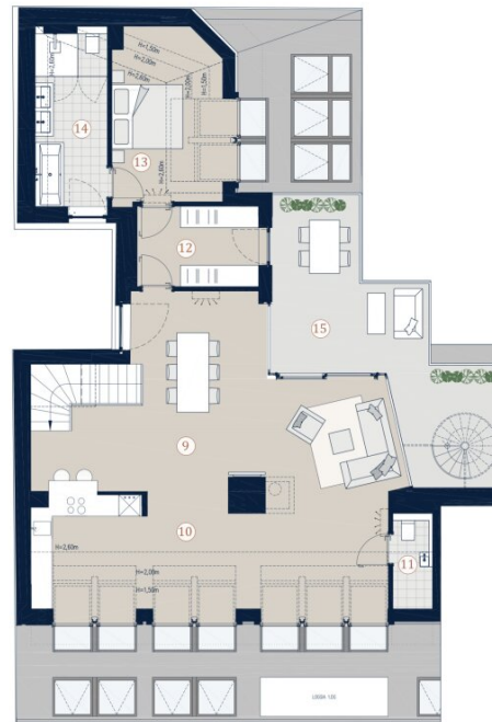
2. Dachgeschoß
