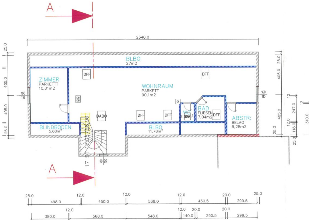
Dachgeschoß
