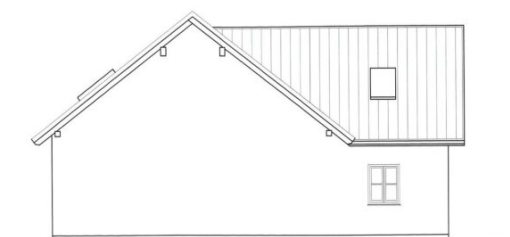
ANSICHT NORD-WEST
