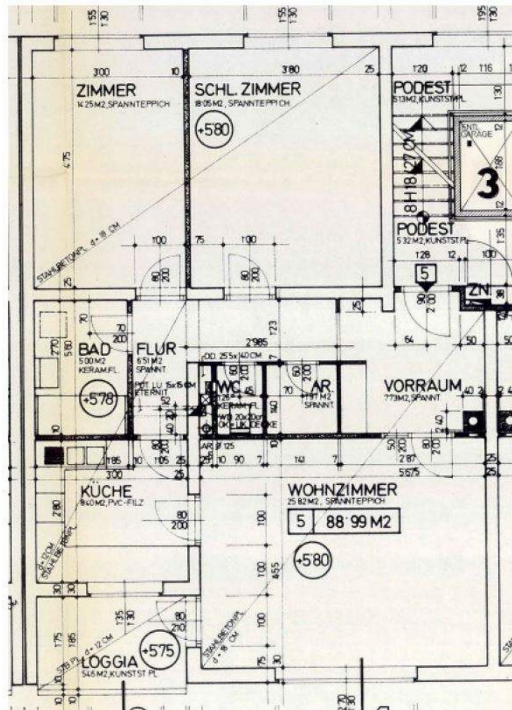
Grundriss
