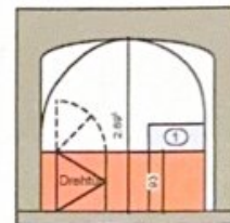
Schnitt A-A
