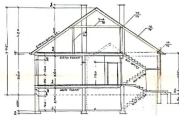
SCHNITT A-B
