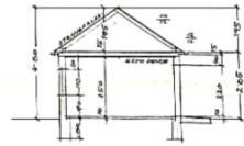
SCHNITT C-D
