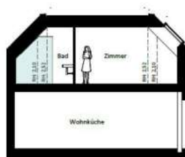
SCHNITT H 03
