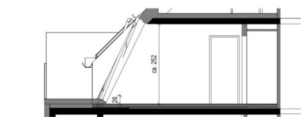
Schnitt 48.A
