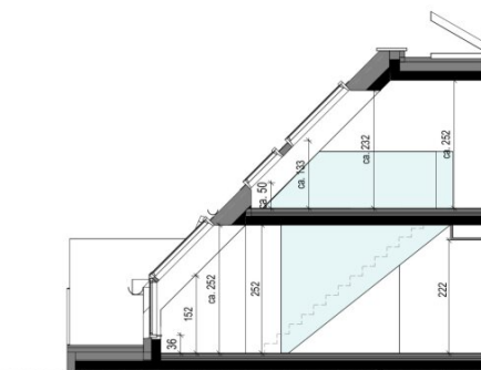
Schnitt 48.B
