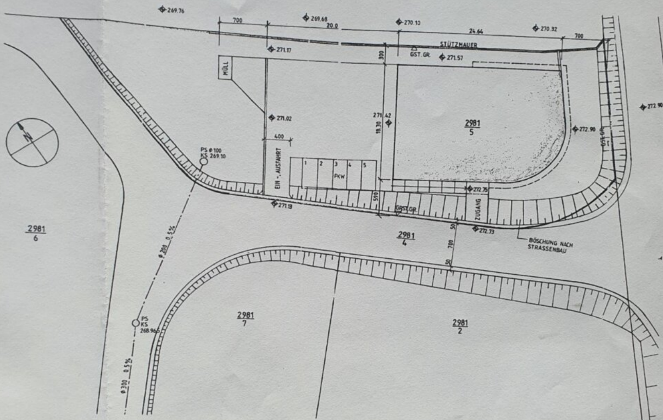
LAGEPLAN
