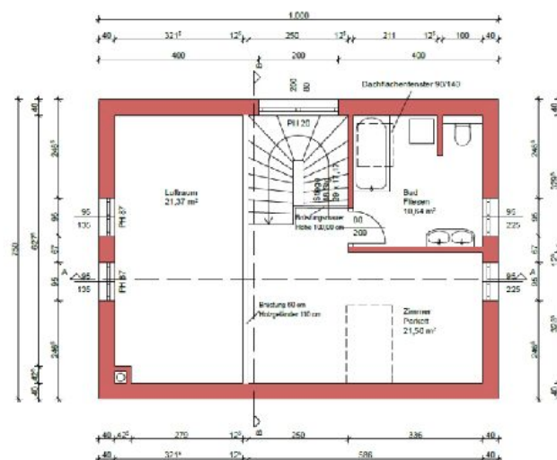
OBERGESCHOSS HAUS 2
