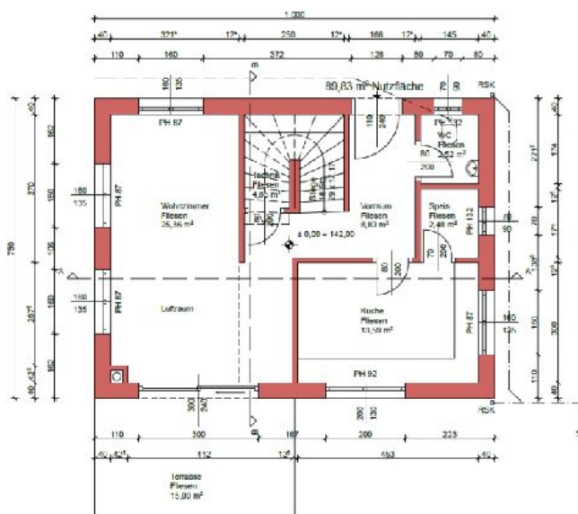
ERDGESCHOSS HAUS 2
