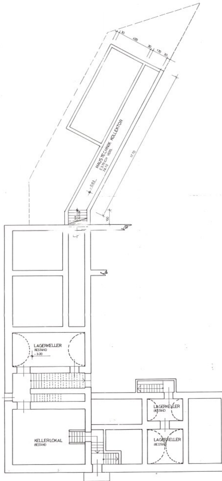
GRUNDRISS KELLERGEŠCHOSS
