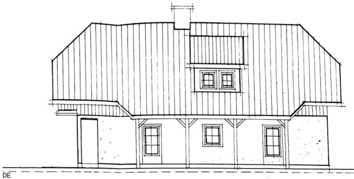
SÜDANSICHT
