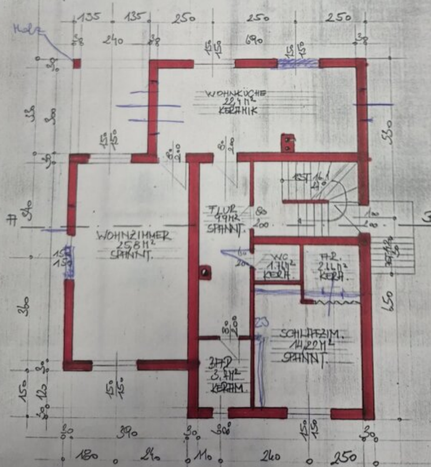
ERDGESCHOSS
