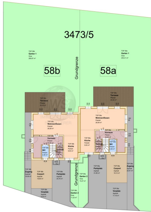
0. Endgeschoss 1:100
