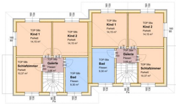
1. Obergeschoss 1:100
