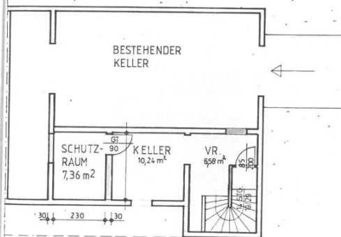
BESTEHENDES KELLERGEOSCHOSS
