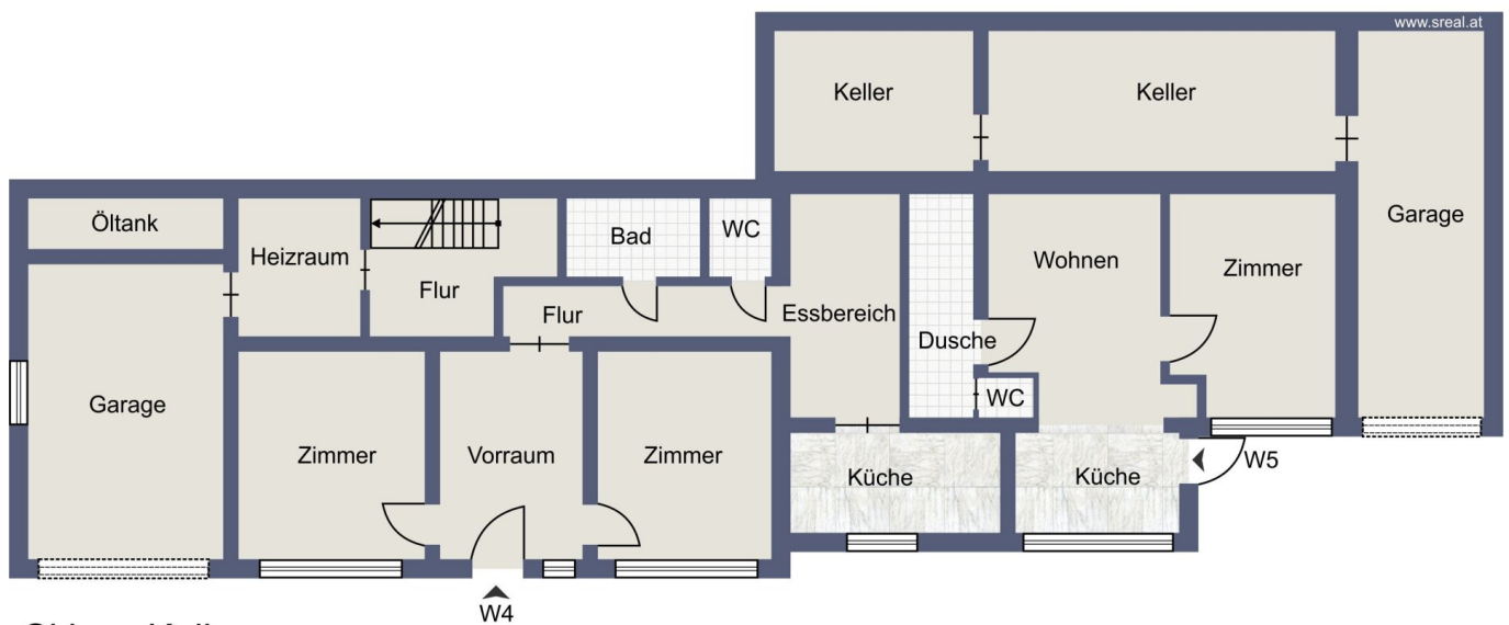
Skizze Keller
