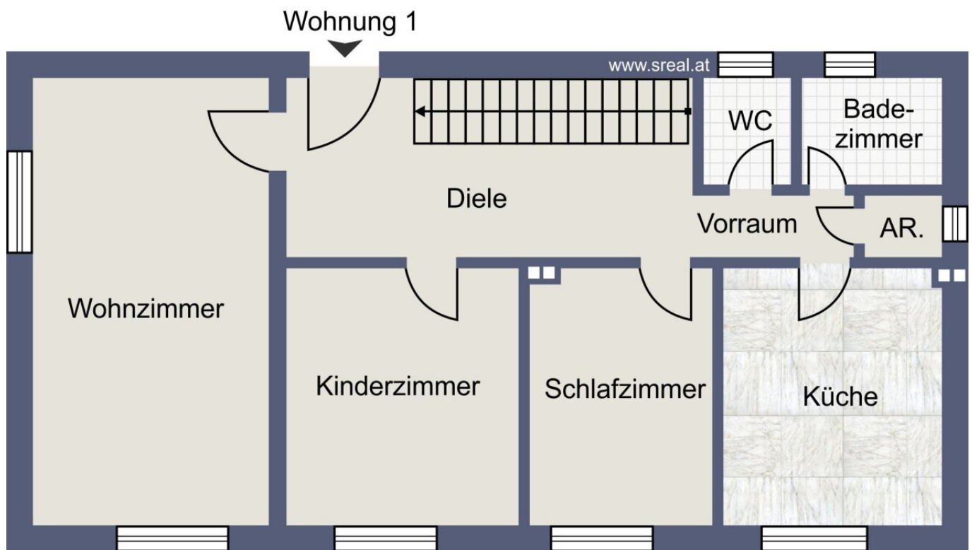
Skizze Obergeschoss
