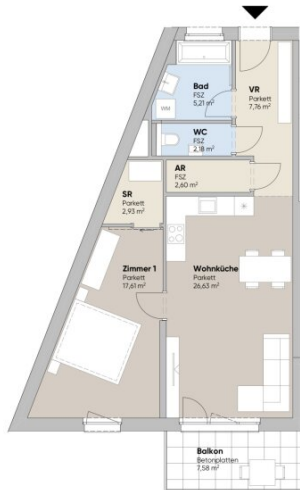
1. Obergeschoss
