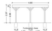
ANSICHT WEST/OST M1:100
