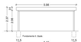
ANSICHT NORD/SÜD M1:100
