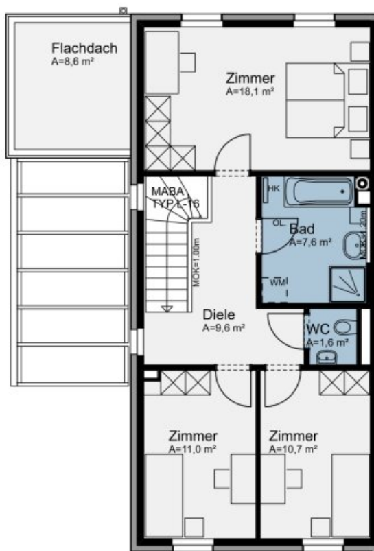
Obergeschoss
