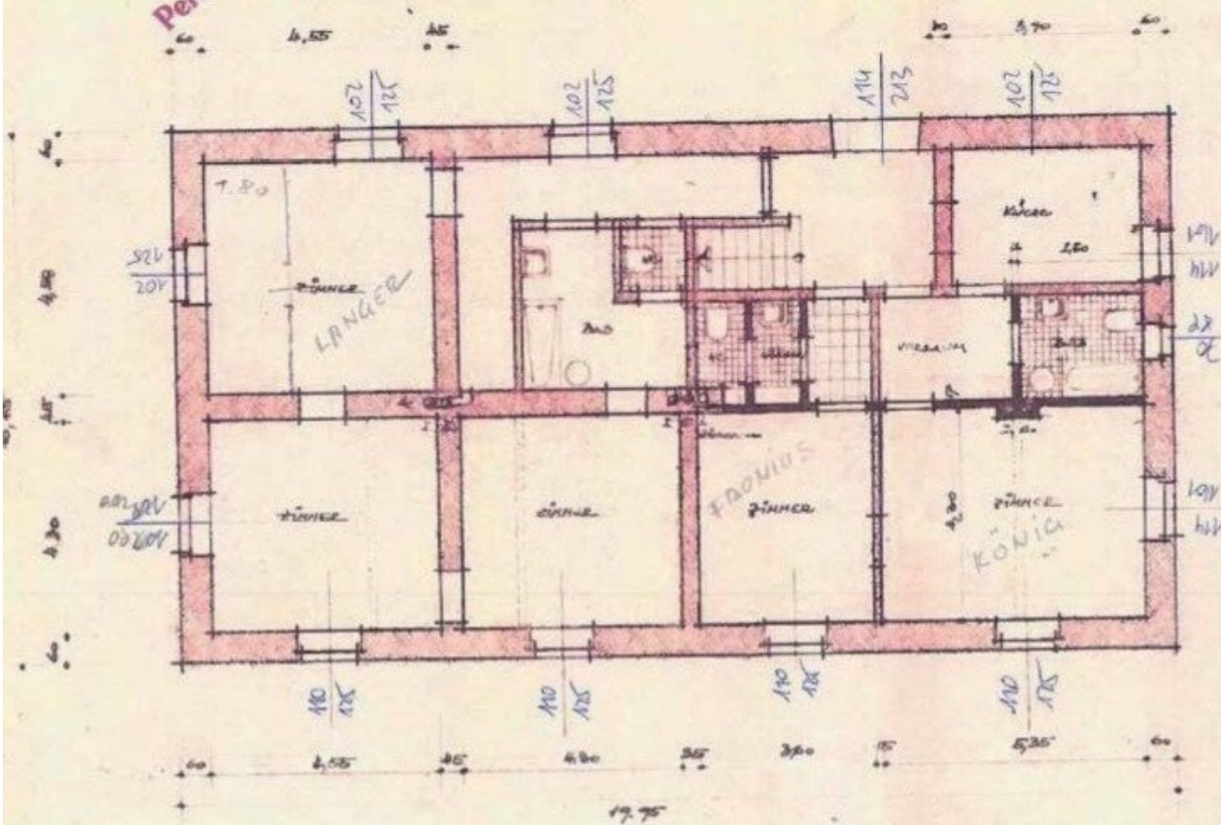
GRUNDRISS GEBÄUDE 12.00
