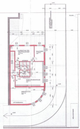
1. OBERGESCHOSS
