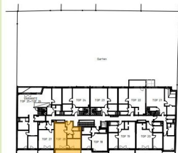
ÜBERSICHTSPLAN 2.OG
