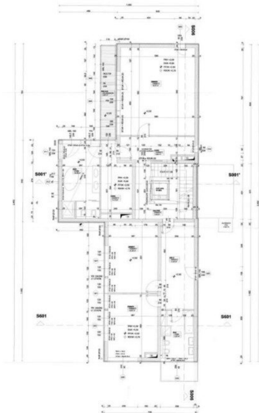
1. Obergeschoß
