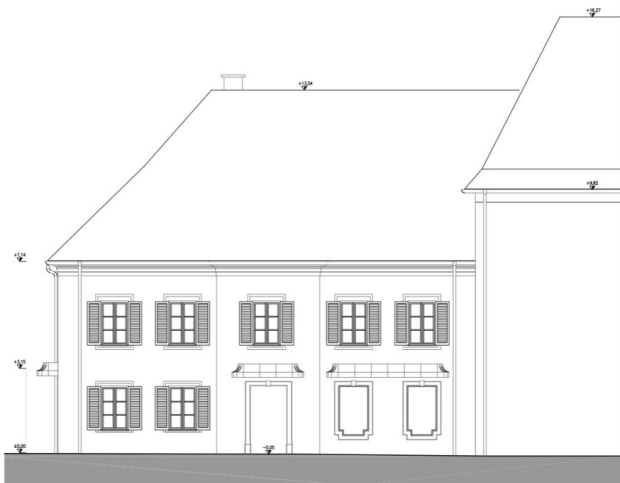
ANSICHT WEST M1:100
