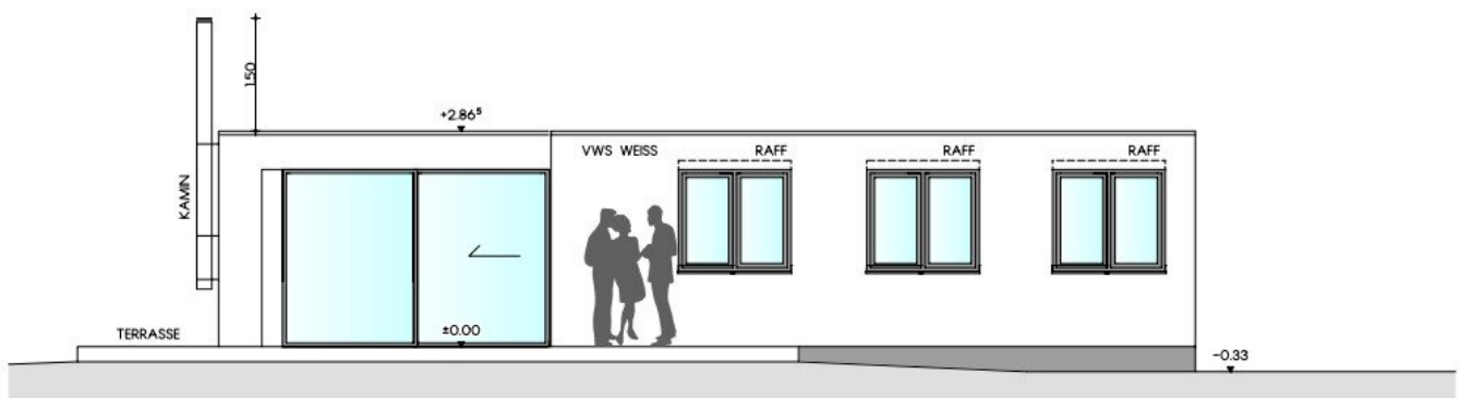
SÜDANSICHT
