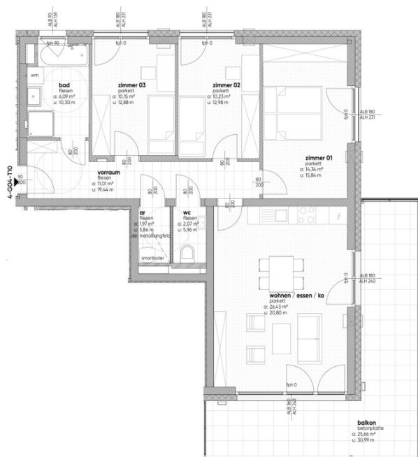
grundriss M 1:75
