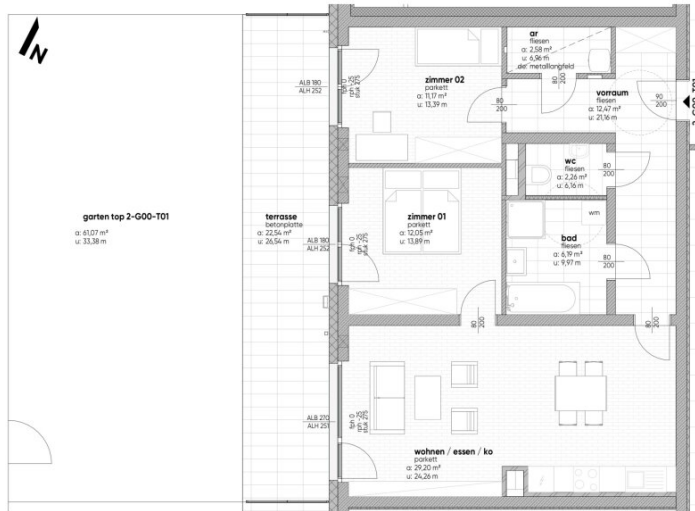
grundriss M 1:75
