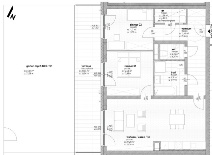
grundriss M1:75
