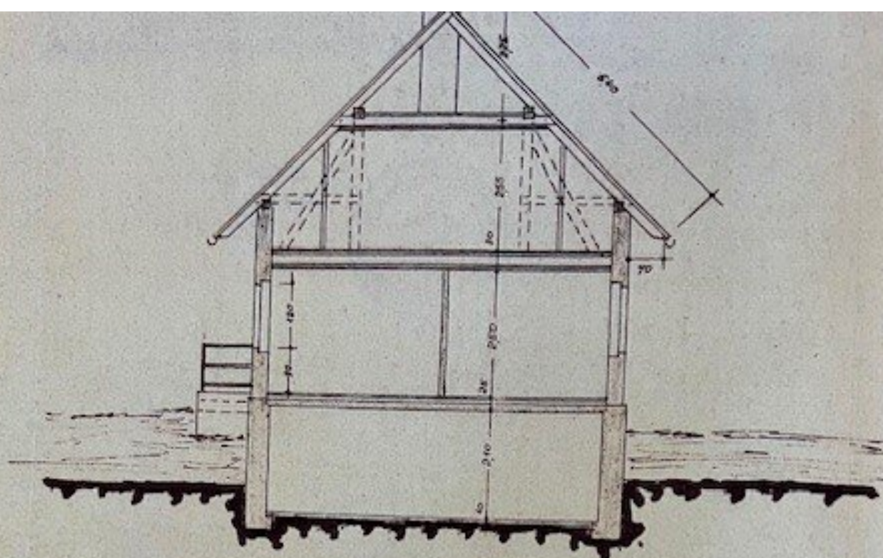
SCHNITT
