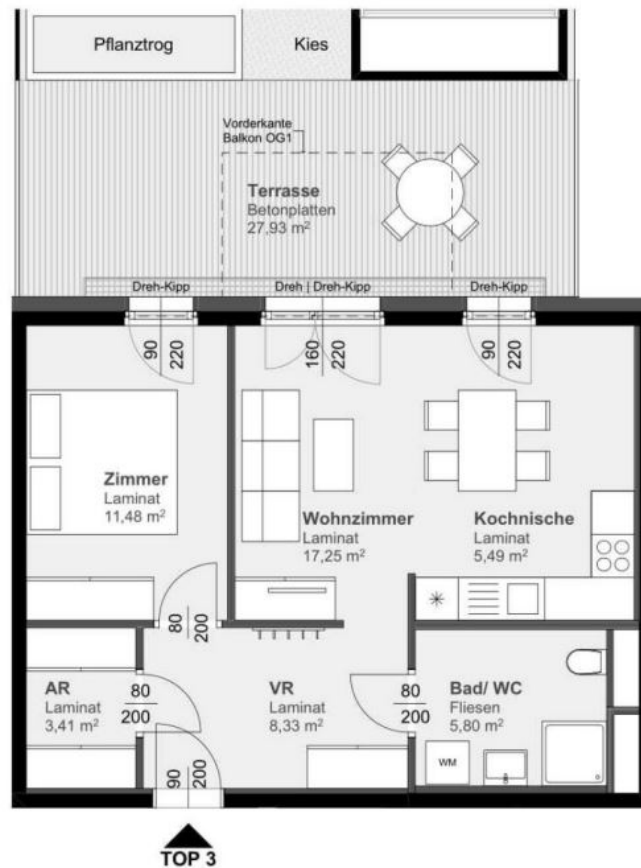
Grundriss Top 3
