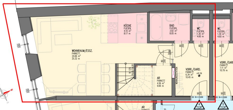
Grundriss 2.OG M= 1:50
