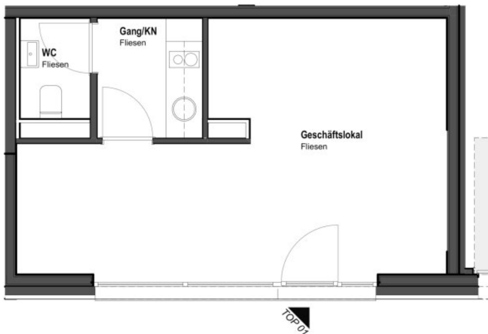
Grundriss 1:50
