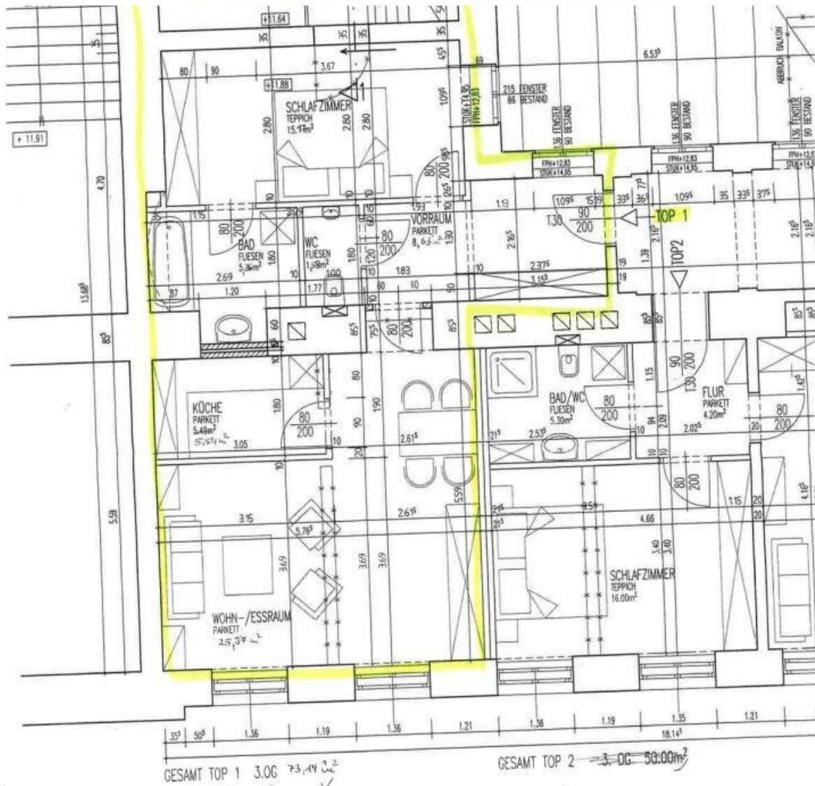
GRUNDRISS 3. OBERGESCHOSS
