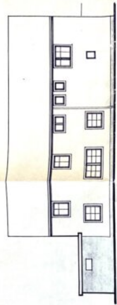
SÜDANSICHT
