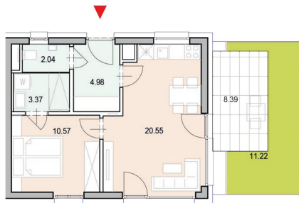
TOP 10 - ERDGESCHOSS WOHNNUTZFLÄCHE 41,51 m²
