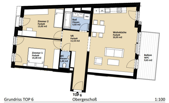
Grundriss TOP 6
