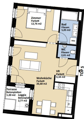
Grundriss TOP 5 Obergeschoß 1:100
