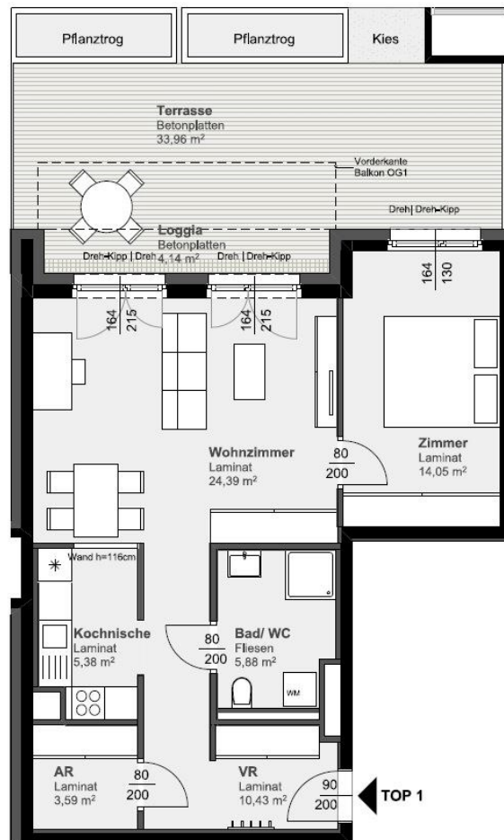
Grundriss
