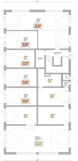
ERDGESCHOSS 1:100
